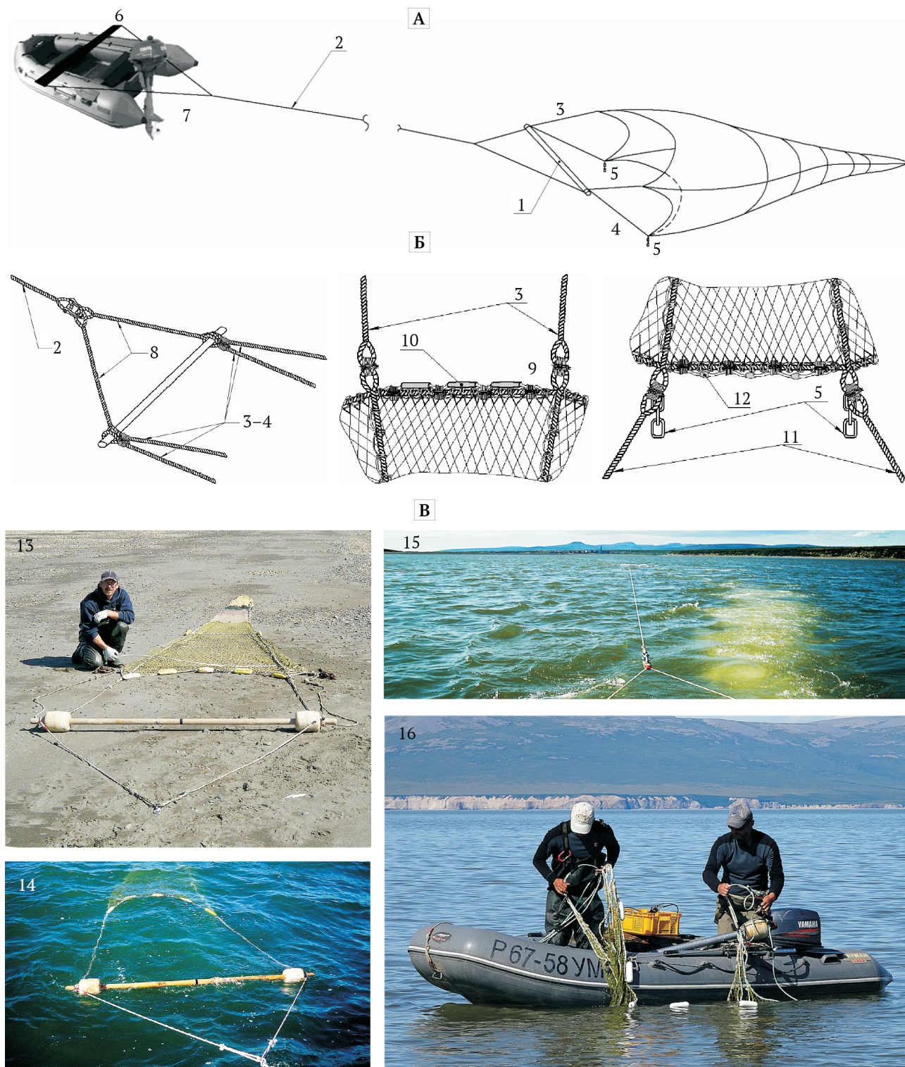
Рис. 4. Бим-трал 8,2×2,0 м для контрольного лова молоди рыб в пелагиали (А — схема траловой системы. Б — основные элементы оснастки трала: 1 — бим; 2 — ваер; 3 — верхний кабель; 4 — нижний кабель; 5 — груз-углубитель; 6 — буксировочная доска; 7 — буксировочные оттяжки; 8 — уздечки; 9 — верхняя подбора; 10 — наплава; 11 — нижняя подбора; 12 — грузила. В — примеры работы с тралом: 13 — р. Камчатка, июль 2010 г.; 14 — прибрежные воды Охотского моря в районе устья р. Хайрюзова, август 2012 г.; 15 — устьевая область р. Пенжины, август 2014 г.; 16 — Пенжинская губа, август 2015 г.) Fig. 4. Beam-trawl 8.2×2.0 m for the control fishing of juvenile fish in the pelagial (A — scheme of the trawl system. B — basic elements of the trawl equipment: 1 — beam; 2 — wire; 3 — headrope; 4 — footrope; 5 — wire load; 6 — trawl door; 7 — towing sweeps; 8 — bridles; 9 — top panel; 10 — floats; 11 — bottom panel; 12 — sinkers. B — examples of the work with the trawl: 13 — Kamchatka R., July 2010; 14 — coastal waters of the Sea of Okhotsk near the Khairyzova R. mouth, August 2012; 15 — mouth of Penzhina R., August 2014; 16 — coastal waters of the Sea of Okhotsk near the Penzhina R. mouth, August 2015)
