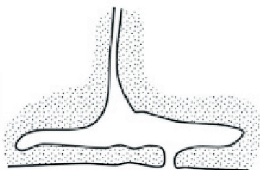
Эстуарная лагуна Estuarine lagoon
