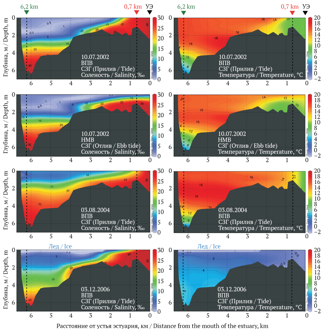
Рис. 36. Продольное распределение солёности (‰) и температуры (°C) воды в эстуарии р. Большой Вилуй (от его устья до кутовой части оз. Бол. Вилуй) в отдельные периоды 2002, 2004 и 2006 г. (по материалам из: Горин, 2013б). Условные обозначения те же, что и на рис. 33; УЭ — устье эстуария Fig. 36. The longitudinal distribution of water salinity (‰) and temperature (°C) in the estuary of the Bolshoi Vilyui River (from the mouth to the pot of Bolshoi Vilyui Lake) in some periods in 2002, 2004 and 2006 (based on materials from Горин, 2013б). Symbols are the same as in Fig. 33; УЭ — estuary mouth
