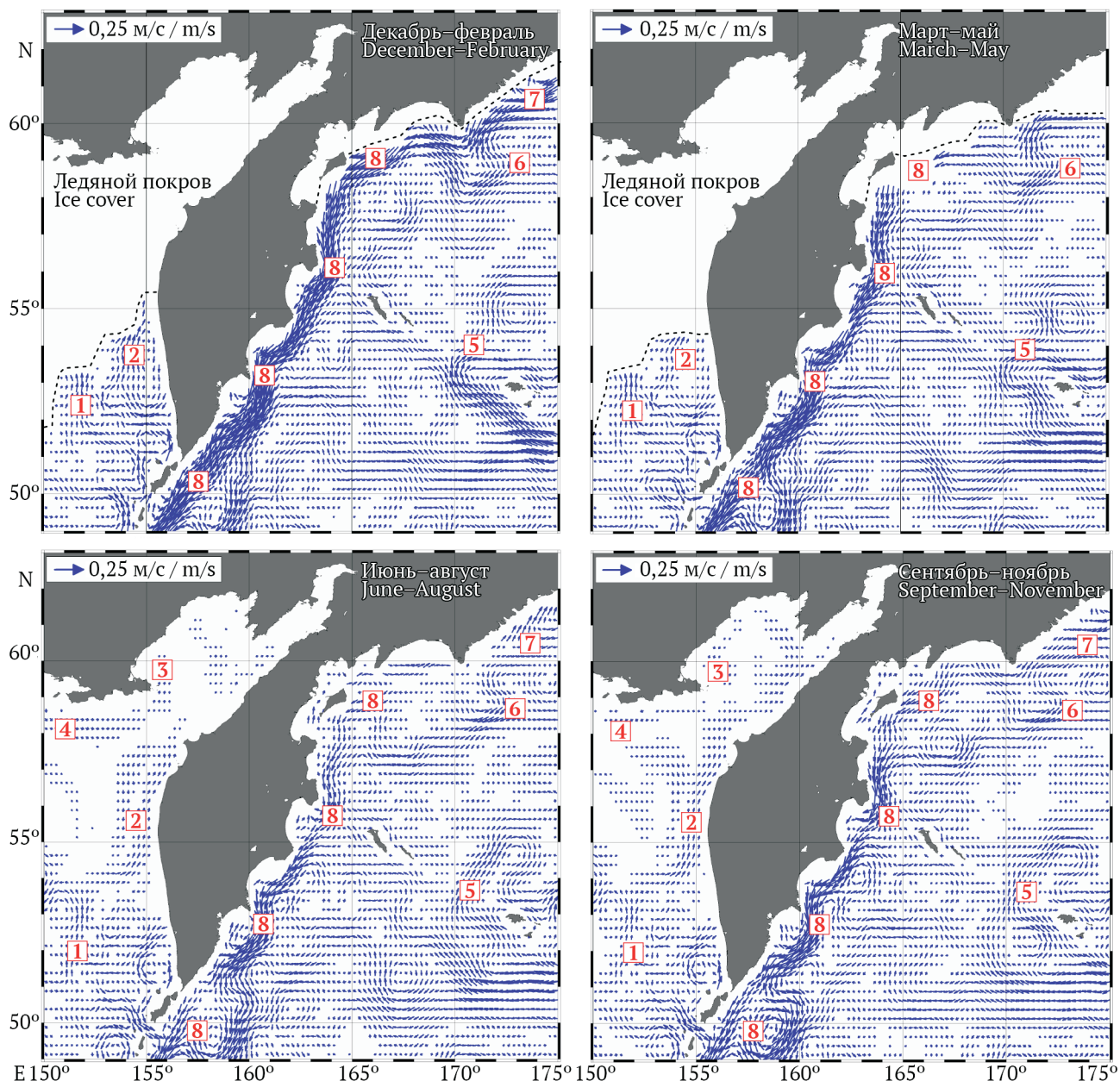
Рис. 25. Распределение направления и скорости течений на поверхности у побережья Камчатки в различные сезоны года (по осредненным данным альтиметрических наблюдений за период с января 1993 по декабрь 2019 г.; источник: www.marine.copernicus.eu ). Условные обозначения течений: 1 – Срединное, 2 – Западно-Камчатское, 3 – Ямское, 4 – Северо-Охотское, 5 – Атту, 6 – Поперечное, 7 – Наваринское, 8 – Камчатское
