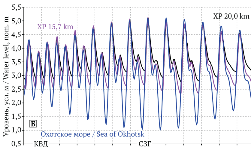
Рис. 32. Пространственно-временные изменения основных гидрологических характеристик в макроприливном русловом эстуарии рр. Хайрюзова–Белоголовая в октябре 2011 г. (по данным стационарных гидрологических наблюдений): А – схема эстуария (условные обозначения: 1 – морская часть; 2 – речные части; МКПО – морской край приливной осушки; УСР – устьевой створ реки; ПрО – приливная осушка; XP – р. Хайрюзова; БГ – р. Белоголовая); Б–Г – колебания уровня (Б, усл. м), солёности (Б, ‰) и температуры (Г, °С) воды у дна Fig. 32. Spatial and temporal changes of the main hydrological characteristics in the macrotidal channel estuary of the Khairyuzova–Belogolovaya rivers in October 2011 (based on stationary observations): А – the scheme of the estuary (The symbols: 1 – marine part; 2 – river parts; МКПО – the marine edge of tidal flat; УСР – the river mouth; ПрО – the tidal flat; XP – Khairyuzova R.; БГ – Belogolovaya R.); Б–Г – the fluctuations of water level (Б, nominal m), salinity (Б, ‰) and temperature (I, °C) near the bottom
