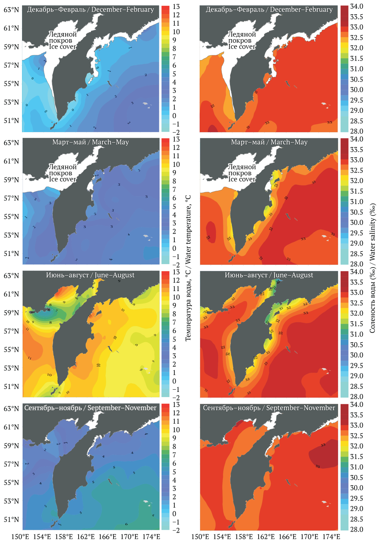
Рис. 26. Пространственное распределение температуры (°C, лев. рис.) и солёности (‰, прав. рис.) воды на поверхности у побережья Камчатки в различные сезоны года (по осредненным данным прямых гидрологических наблюдений за период с 1955 по 2013 г.; источник: https://www.nodc.noaa.gov/OC5/woa13/ ). Также приведена средняя площадь акватории, покрытой морским льдом за период с января 2006 по декабрь 2019 г.; источник: https://nsidc.org/ Fig. 26. Spatial distribution of surface water temperature (°C, left fig.) and salinity (‰, right fig.) off the Kamchatka coast in different seasons of the year (based on averaged data hydrological observations in situ for the period from 1955 to 2013; data source: https://www.nodc.noaa.gov/OC5/woa13/ ). The figures also show the average area of water area covered by sea ice for the period from January 2006 to December 2019; data source: https://nsidc.org/
