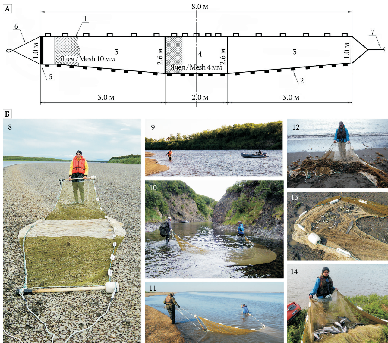
Рис. 5. Закидной невод 8,0×2,6 м для контрольного лова рыб на литорали (А — сборочный чертеж с основными элементами невода: 1 — верхняя подбора с наплавами; 2 — нижняя подбора с грузами; 3 — крылья; 4 — сливная часть; 5 — кляч; 6 — уздечка; 7 — урез. Б — примеры работы с неводом: 8 — р. Таловка, август 2014 г.; 9 — р. Белоголовая, июль 2012 г., 10 — р. Ловаты, северная часть Пенжинской губы, июль 2015 г.; 11 — устье р. Ича, июнь, 2018 г.; 12 — бух. Вилучинская, июнь 2019 г.; 13–14 — р. Вывенка, июль 2021 и 2022 г.) Fig. 5. Beach seine 8.0×2.6 m for the control fishing on the littoral (A — assembly drawing with the main elements of the seine: 1 — headrope with floats; 2 — footrope with weights; 3 — wings; 4 — drainage part; 5 — lead end; 6 — bridle; 7 — warp. Б — examples of the work with the seine: 8 — Talovka R., August 2014; 9 — Belogolovaya R., July 2012; 10 — Lovaty R., northern part of Penzhina Bay, July 2015; 11 — the Icha R. mouth, June, 2018; 12 — Vilyuchinskaya Bay, June, 2019; 13–14 — Vyvenka R., July, 2021 and 2022)
