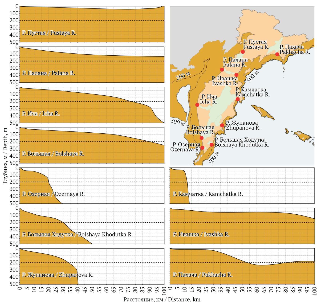
Рис. 23. Карта глубин и батиметрические профили подводного берегового склона (до глубины 500 м и на дистанции 100 км от берега) в районе устьев некоторых рек, расположенных на восточном и западном побережье Камчатки Fig. 23. Depth map and bathymetric profiles of the underwater coastal slope (to a depth of 500 m and at a distance of 100 km from the shore) near of some river mouths located on the eastern and western coasts of Kamchatka
