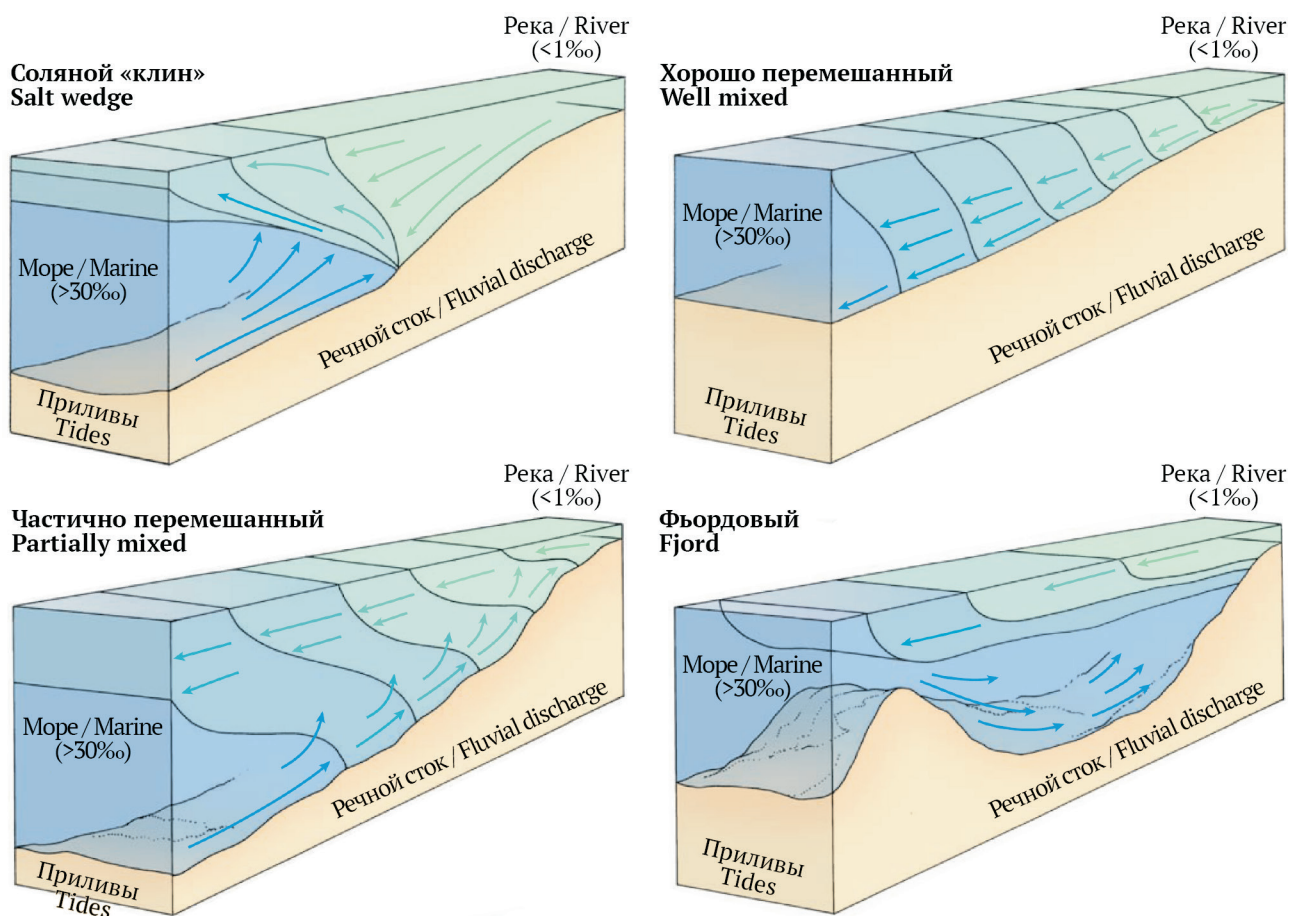
Рис. 29. Пример классификации эстуариев по продольному распределению солености воды (по: Cameron, Pritchard, 1963; Valle-Levinson, 2010; Karleskint et al., 2010) Fig. 29. Example of classification of estuaries based on water salinity longitudinal distribution (based on Cameron and Pritchard, 1963; Valle-Levinson, 2010; Karleskint et al., 2010)
