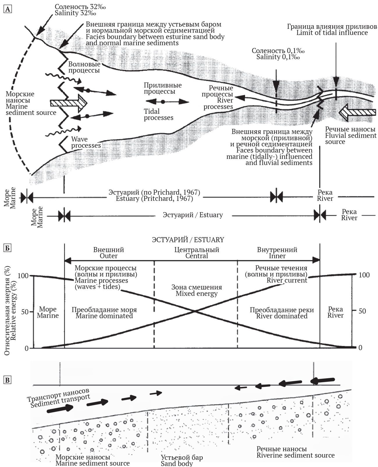
Рис. 11. Схематическое изображение основных гидролого-морфологических устьевых процессов, действующих в типичных эстуариях (А), результирующая трехсторонняя зональность границ (Б), а также обобщенная схема переноса донного материала (В). Внутренняя «речная» граница эстуария в соответствии с представленной схемой почти всегда проходит на суше от значения солености 0,1‰, однако внешняя «морская» граница может проходить как по суше (как показано на этом рисунке), так и по морю до значений солености воды до ~32‰ (по данным Dalrymple et al., 1992). Fig. 11. Schematic representation of the main hydrologic-morphological processes in typical estuaries (A), generalized three-dimensional boundaries (B) and scheme of bottom material movement (B). According to the presented scheme, the inner "river" boundary of estuary is almost invariably on land at salinity 0,1‰, while the outer "marine" boundary can be either on land (as shown in this figure) or offshore at salinities \leq 32‰ (based on Dalrymple et al., 1992).
