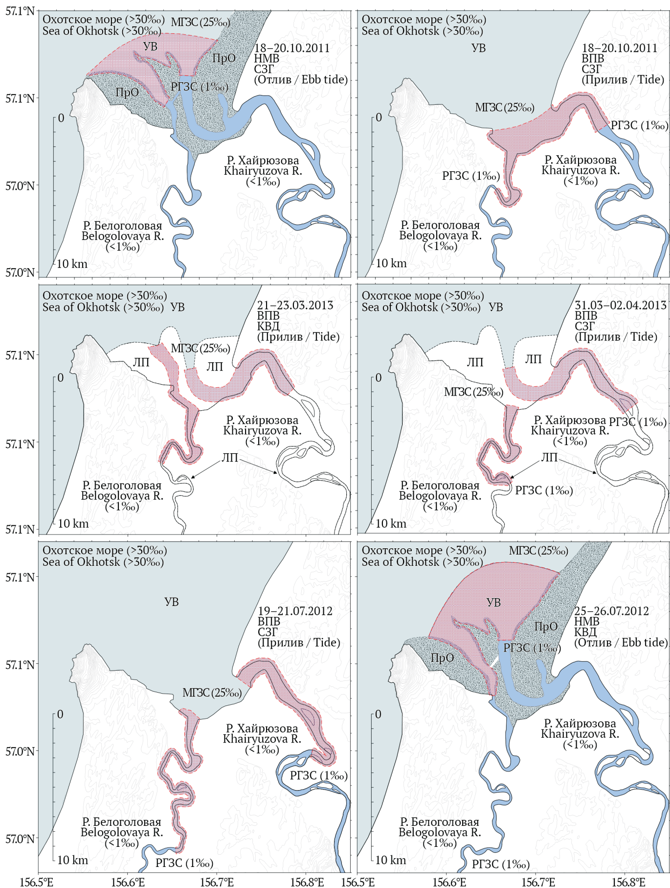
Рис. 57. Примеры расположения зоны смешения (ЗС) в макроприливном воронкообразном эстуарии рек Хайрюзова и Белоголовая в различные сезоны 2011–2013 гг. Условные обозначения: МГЗС – условно-морская граница ЗС по предельному положению изогалины 25‰ в поверхностном горизонте; РГЗС – условно-речная граница ЗС по предельному положению изогалины 1‰ в придонном горизонте; УВ – устьевое взморье; ПрО – приливная осушка; ЛП – ледяной покров; ВПВ – высокие полные воды; НМВ – низкие малые воды; СЗГ – сизигийный прилив; КВД – квадратурный прилив (по: Горин и др., 2012; Коваль и др., 2012; Горин, Коваль, 2014) Fig. 57. Examples of mixing zone (ЗС) location within the macrotidal channel estuary with mouth widening of Khairuzova and Belogolovaya rivers in different seasons of 2011–2013 (The symbols: МГЗС – conventional marine boundary of mixing zone based on terminal position of the isohaline 25‰ in the surface horizon; РГЗС – conventional riverine boundary of mixing zone based on terminal position of the isohaline 1‰ in the demersal horizon; УВ – mouth seashore zone; ПрО – tidal flat zone; ЛП – ice cover; ВПВ – high full water; НМВ – low poor water; СЗГ – syzygial tide; КВД – quadrature tide (based on materials: Горин и др., 2012; Коваль и др., 2012; Горин, Коваль, 2014)
